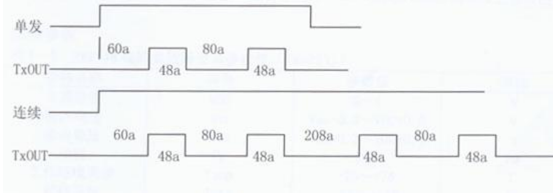
图 1-3 单发和连发输出波形图
